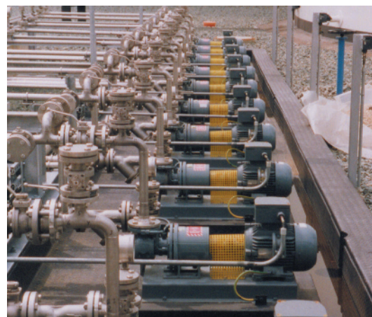
V30-2 STGTRM+Y Liquido trasportato: additivo Pumped fluid: additive - Líquido transportado: aditivo
